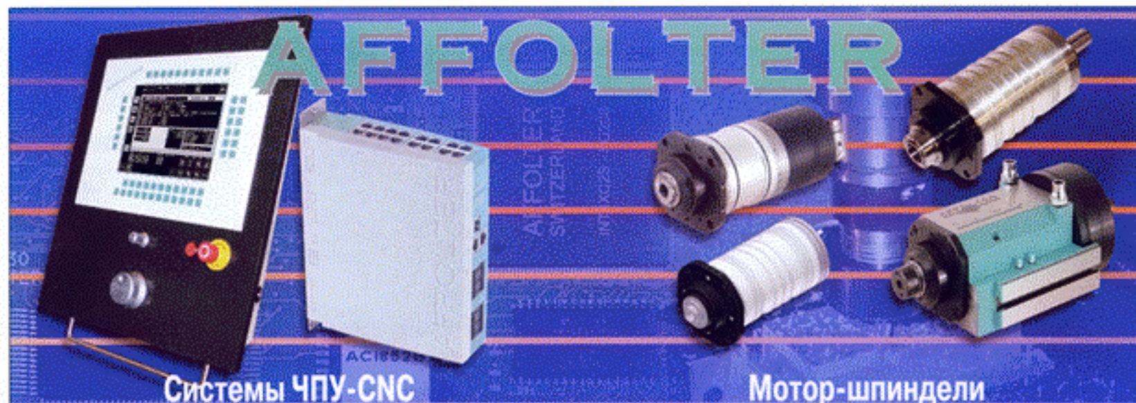
Система ЧПУ типа LESTE 4 с четырьмя ЧПУ-координатами, 16-ю входами и 16-ю выходами (24 В), четырьмя аналоговыми входами и четырьмя аналоговыми выходами, каналами BUS и Ethernet.
